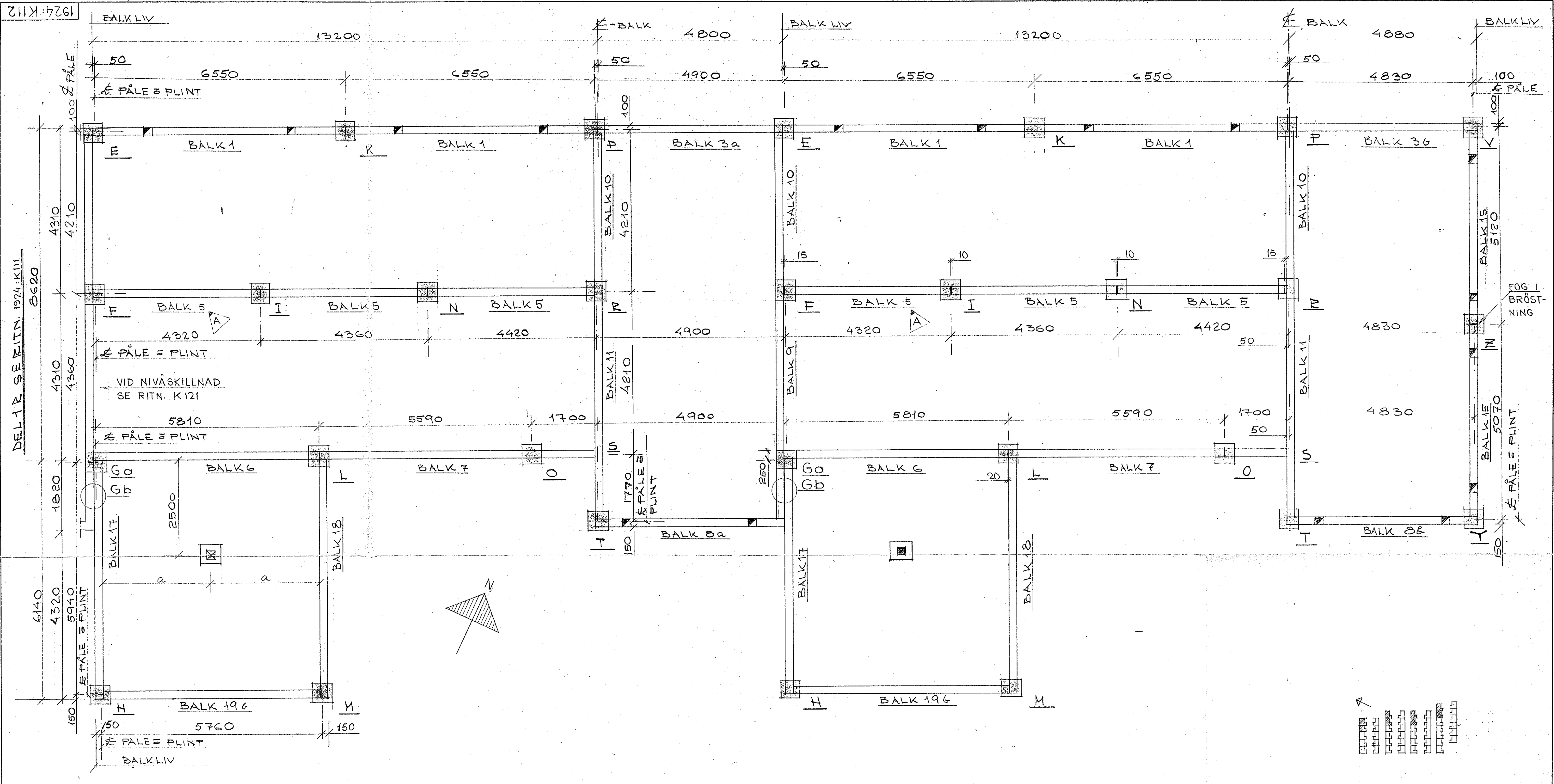
PÅLPLAN 1:50 BETR PÅLNING OCH BETECKNINGAR E-Y SE RITN. 1924:K110
